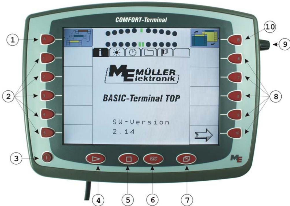
Rys.4-1: Elementy obsługujące COMFORT - Terminal
